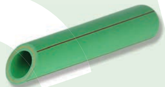
ท่อน้ำร้อนไฟเบอร์ Class: SDR6 PN20 Composite Fibre อุณหภูมิใช้งาน 3 - 95 องศา แรงดันสูงสุด 20 BAR
